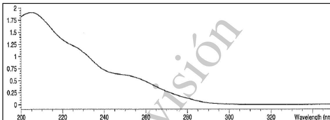
Figura No 5. Espectro guía de identificación de disolución
