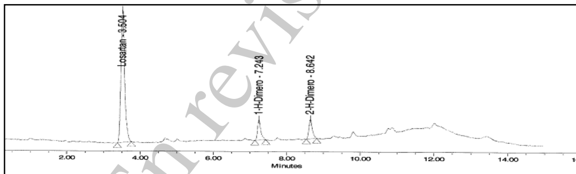
Figura No. 1. Cromatograma guía system suitability valoración losartán
